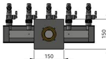
POHLED P
